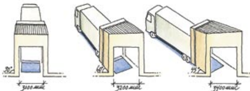
Dimensionering av portar – ett exempel från bokens faktaavsnitt
